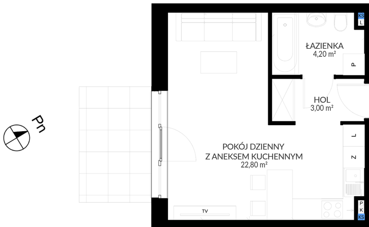
PROPOZYCJA ARANŻACJI MIESZKANIA
